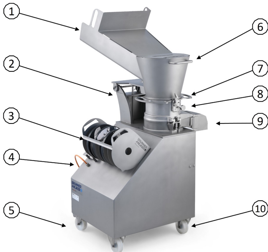
Abb. 3: Aufsatz Trichter
