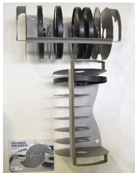
Abb. 41: Wandmontage Schneidscheibenhalter
