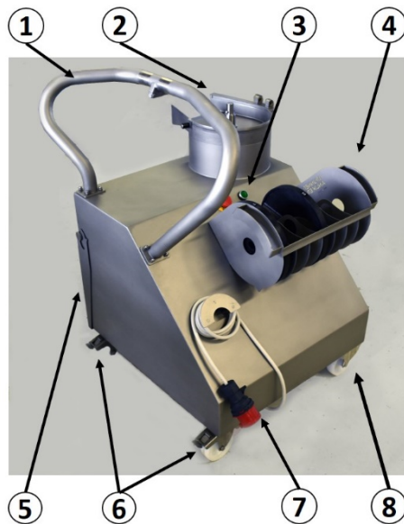
Abb. 2: Systembezeichnung Grundgerät
