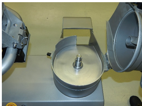
Abb. 20: Trichter und Aufsatzkopf weggeschwenkt
