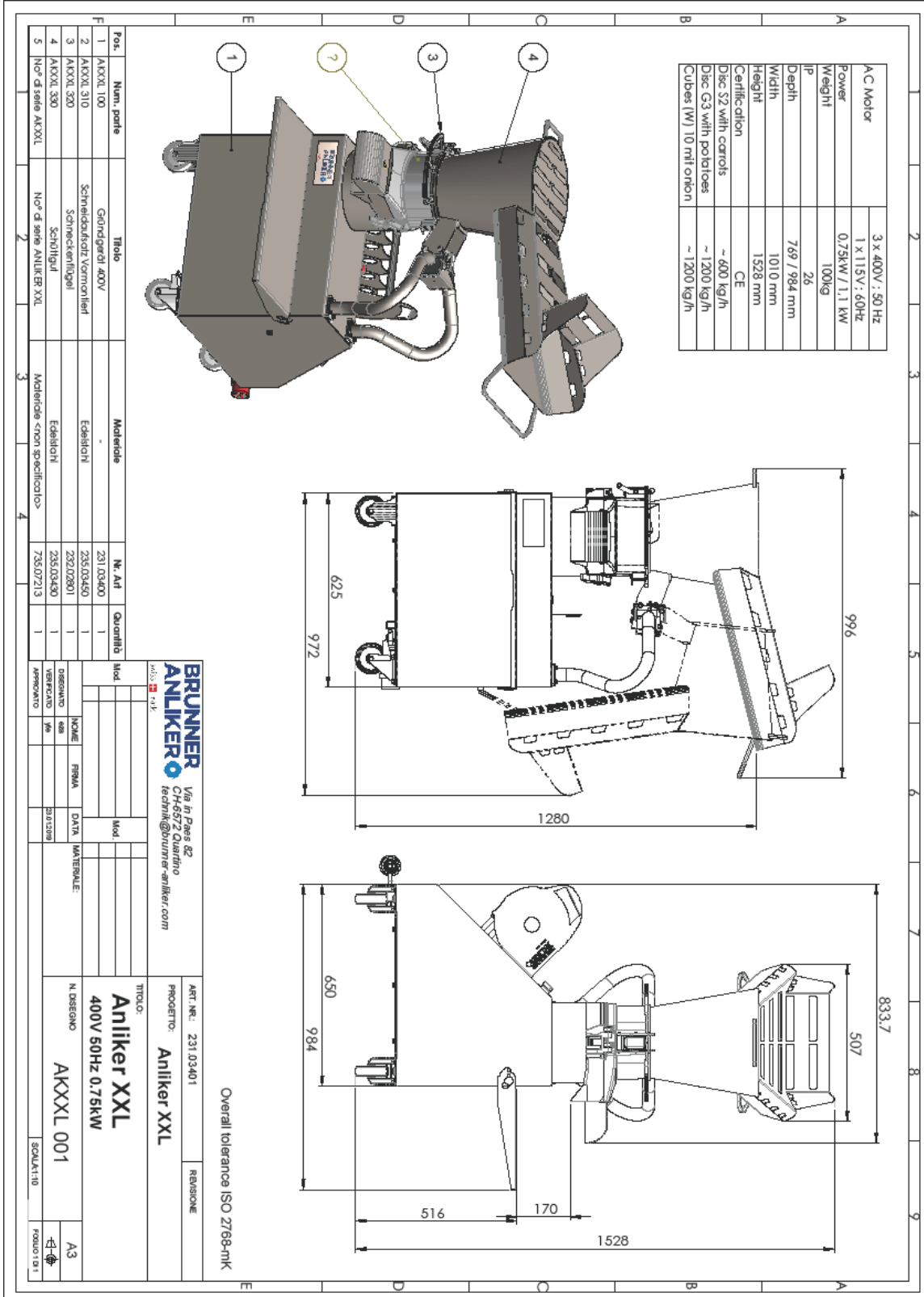
Abb. 33: Massbild ANLIKER XXL
