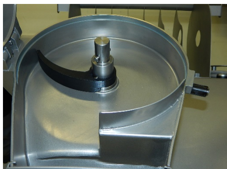
Abb. 21: Auswerfer eingesetzt
