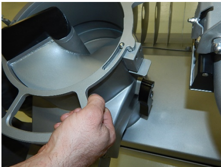
Abb. 23: Schneckenflügel eingesetzt
