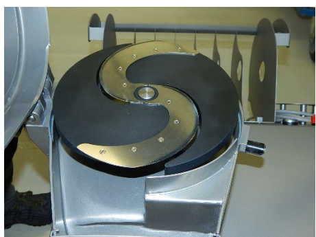
Abb. 22: Schneidscheibe eingesetzt
